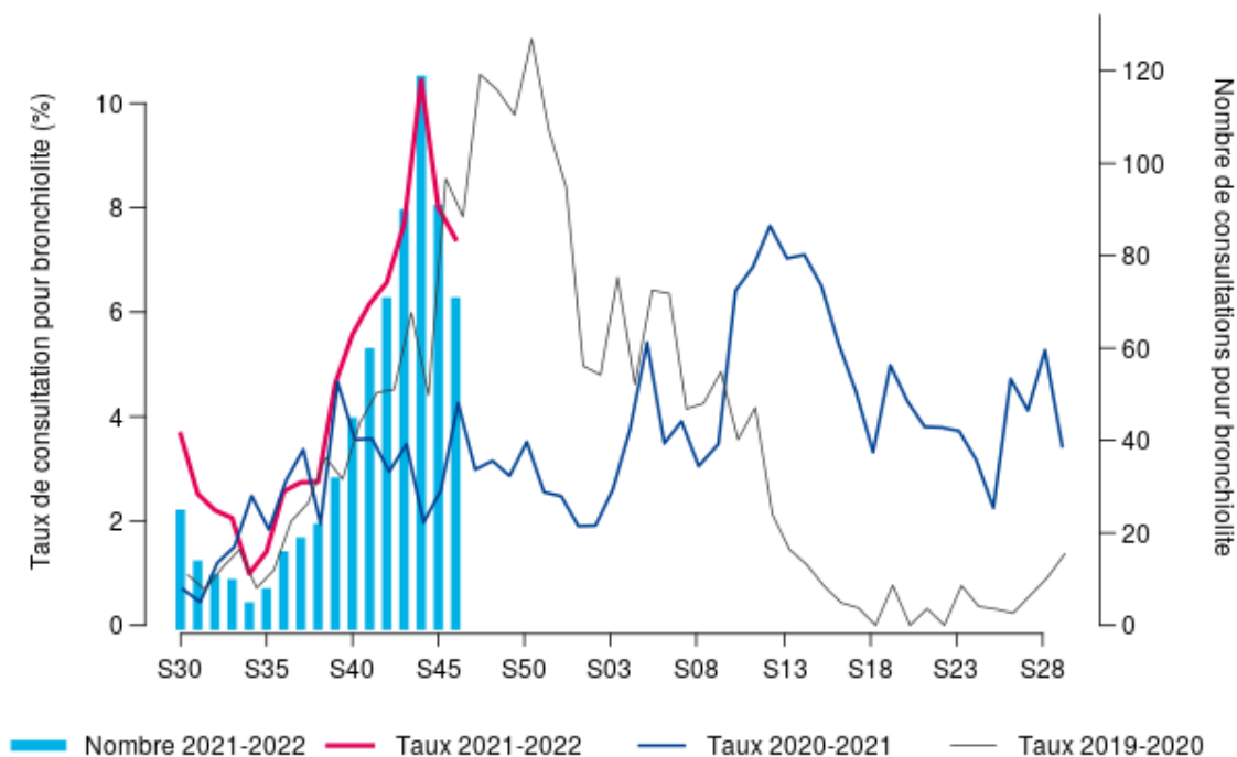
Figure 1. Evolution hebdomadaire du nombre de consultations et proportion d'activité pour bronchiolite chez les moins de 2 ans, SOS Médecins, Nouvelle-Aquitaine ( S47 non disponible )
