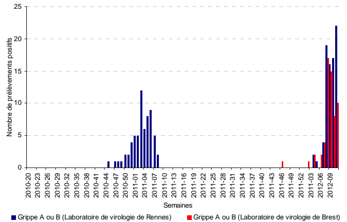
Figure 12 | Evolution hebdomadaire du nombre de virus grippaux de type A ou B isolés parmi les prélèvements respiratoires analysés, tous âges confondus , Laboratoires de virologie des CHU de Rennes (depuis la semaine 2011-11) et Brest (depuis la semaine 2011-43) (Sources : CHU de Rennes et Brest)
