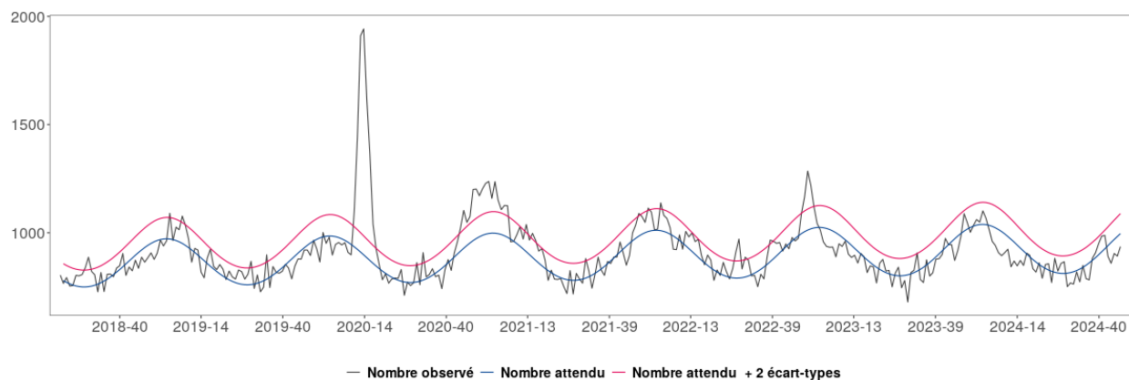
Figure 9. Mortalité toutes causes, toutes classes d'âge confondues, jusqu'à la semaine 47-2024, Grand Est (Source : Insee, au 04/12/2024)
