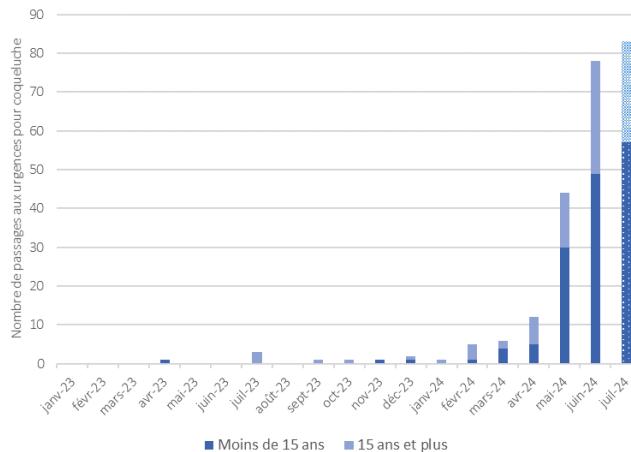
Figure 2. Évolution mensuelle du nombre de passages aux urgences pour suspicion de coqueluche, chez les moins de 15 ans et les 15 ans et plus, Nouvelle-Aquitaine, du 1 er janvier 2023 au 21 juillet 2024 (données non consolidées)
