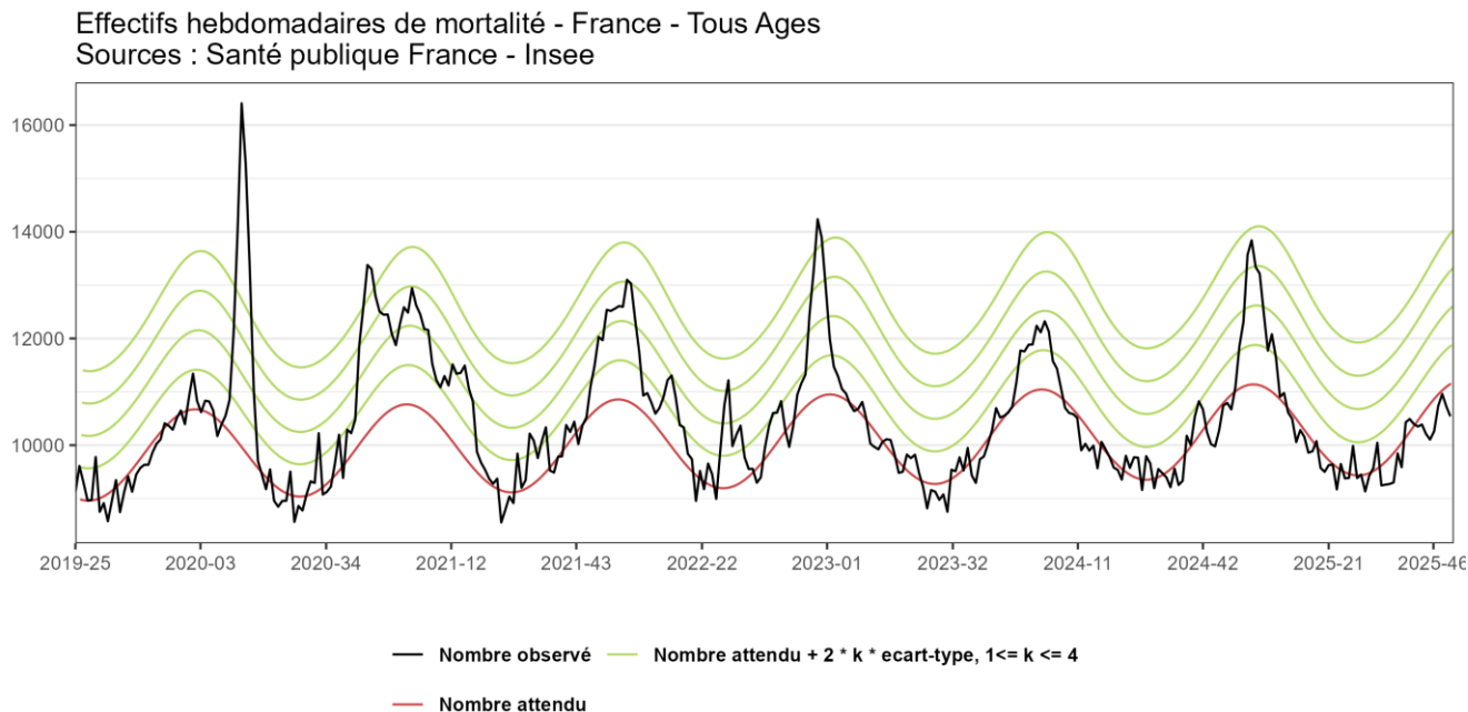
Figure 1 : Fluctuations hebdomadaires des nombres observés (noir) et attendus (rouge) de décès, Tous âges confondus, 2019 à 2025 (jusqu'en semaine 51) - France (Source des données : Insee, actualisation au mardi 30 déc. 2025) (dernière semaine incomplète)
