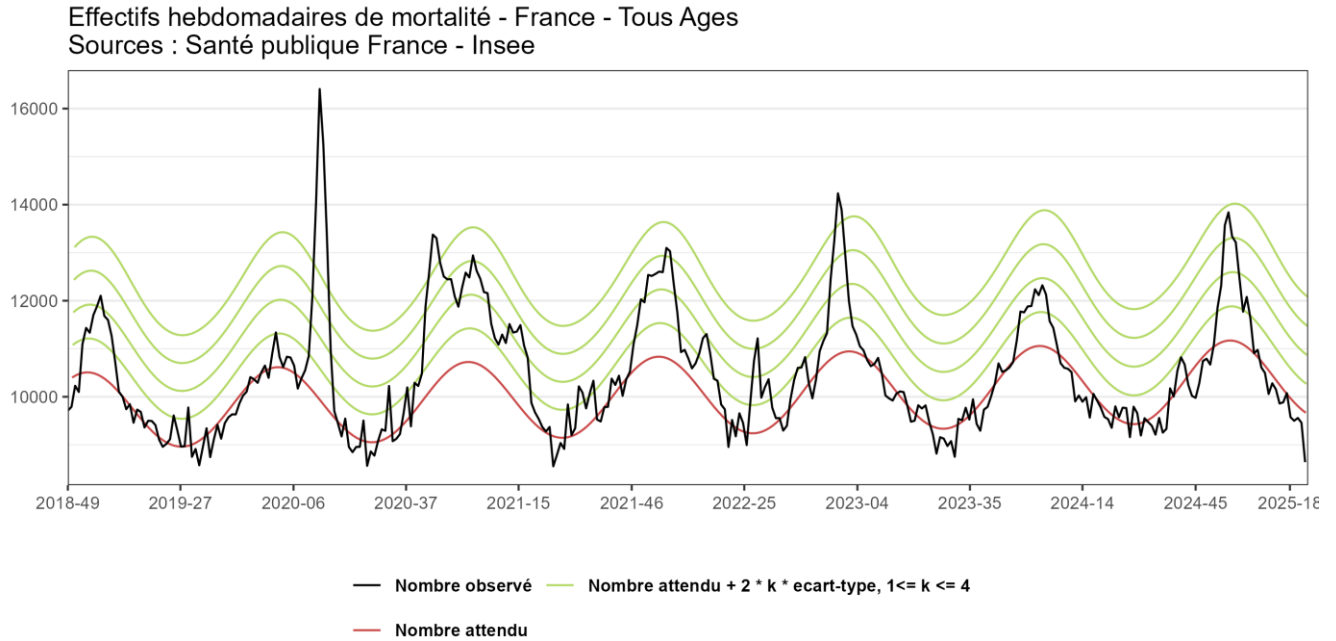
Figure 1 : Fluctuations hebdomadaires des nombres observés (noir) et attendus (rouge) de décès, Tous âges confondus, 2018 à 2024 (jusqu'en semaine 23) - France (Source des données : Insee, actualisation au mardi 17 juin 2025) (dernière semaine incomplète)
