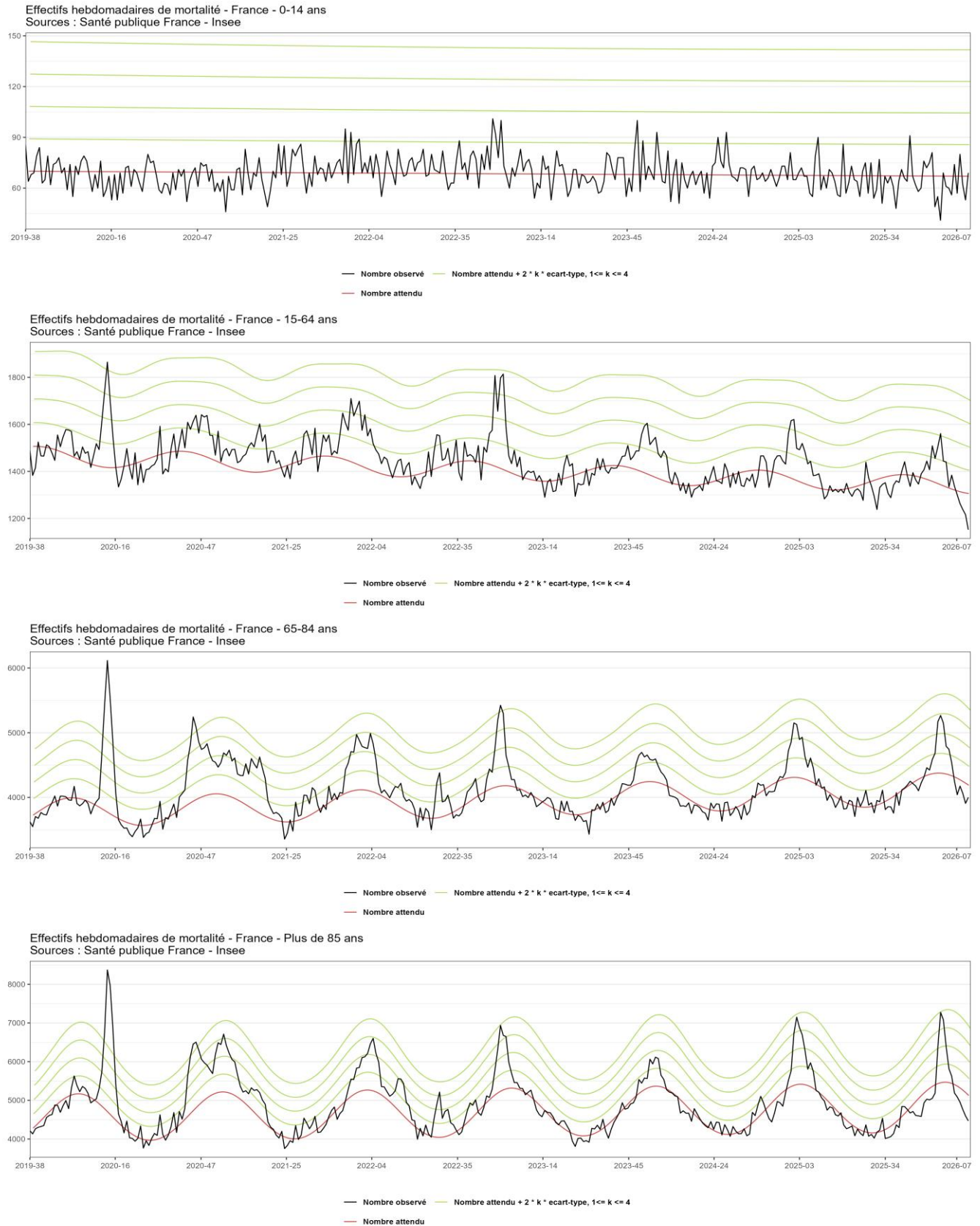
Figure 3 : Fluctuations hebdomadaires de la mortalité par classe d'âges, 2019 à 2026 (jusqu'à la semaine 12) – France (Sources des données : Insee - actualisation au mardi 31 mars 2026)
