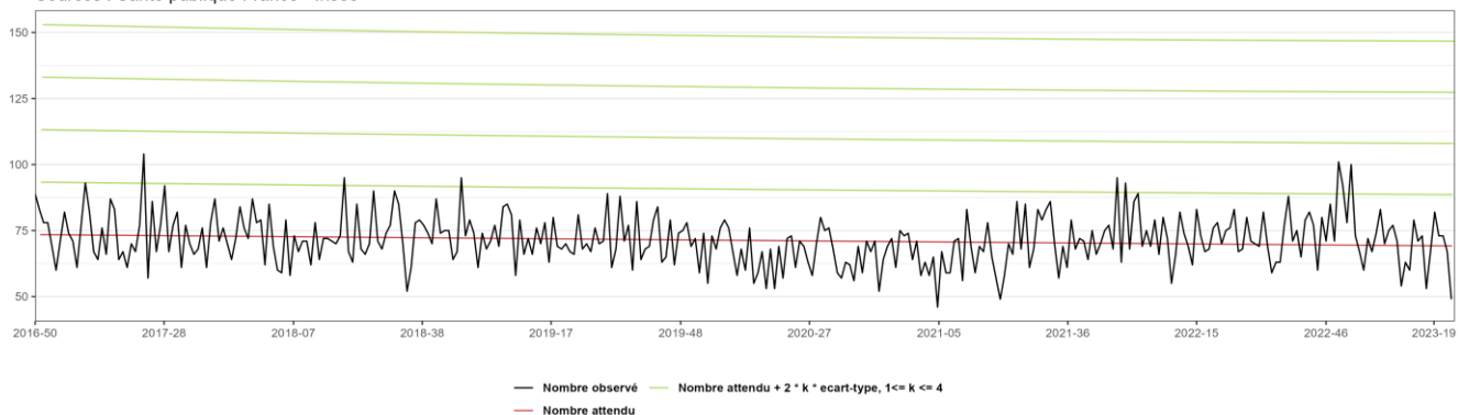
Figure 3 : Fluctuations hebdomadaires de la mortalité par classe d'âges, 2016 à 2023 (jusqu'à la semaine 24) – France (Sources des données : Insee - actualisation au mardi 27 juin 2023)
