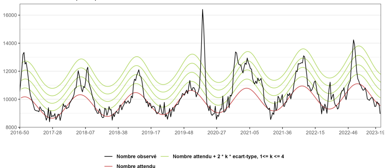
Figure 1 : Fluctuations hebdomadaires des nombres observés (noir) et attendus (rouge) de décès, Tous âges confondus, 2016 à 2023 (jusqu'en semaine 24) - France (Source des données : Insee, actualisation au mardi 27 juin 2023) (dernière semaine incomplète)
