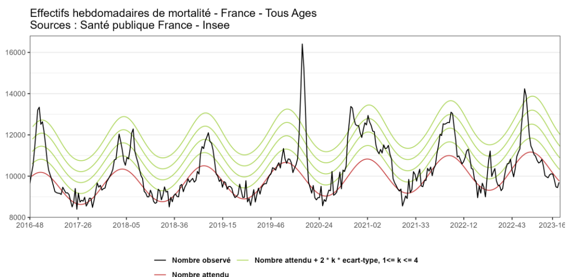
Figure 1 : Fluctuations hebdomadaires des nombres observés (noir) et attendus (rouge) de décès, Tous âges confondus, 2016 à 2023 (jusqu'en semaine 21) - France (Source des données : Insee, actualisation au mardi 13 juin 2023) (dernière semaine incomplète)
