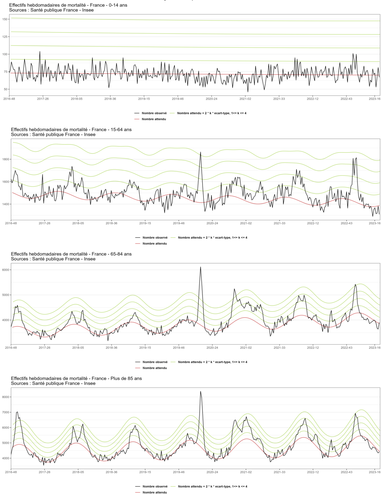
Figure 2 : Fluctuations hebdomadaires de la mortalité par classe d'âges, 2016 à 2023 (jusqu'à la semaine 21) – France
