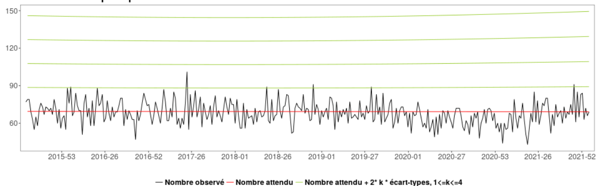
Figure 3 : Fluctuations hebdomadaires de la mortalité par classe d'âges, 2015 à 2022 (jusqu'à la semaine 05) – France (Sources des données : Insee - actualisation au 15 février 2022)
