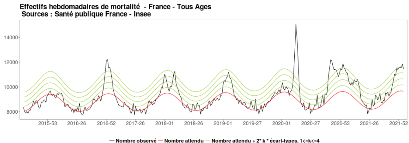
Figure 1 : Fluctuations hebdomadaires des nombres observés (noir) et attendus (rouge) de décès, Tous âges confondus, 2015 à 2022 (jusqu'en semaine 05) - France (Source des données : Insee, actualisation au 15 février 2022) (dernière semaine incomplète)
