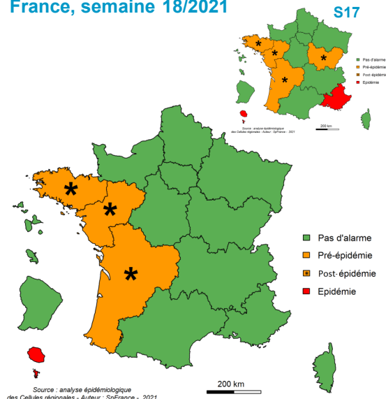
Fig.2-Niveau d'alerte régional de la bronchiolite, enfants de moins de 2 ans, France, semaine 18/2021
