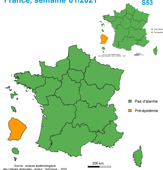
Fig.2-Niveau d'alerte régional de la bronchiolite, enfants de moins de 2 ans, France, semaine 01/2021
