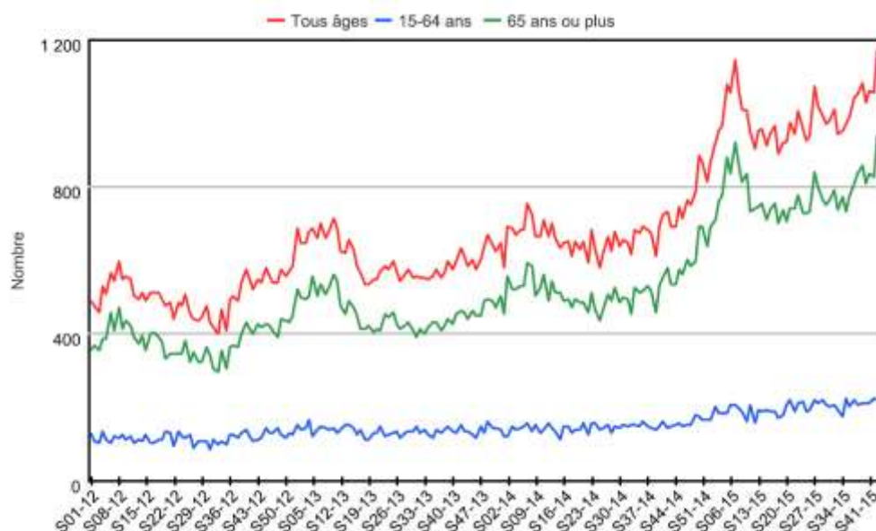
Fluctuations hebdomadaires de la mortalité issue de la certification électronique des décès de 2012 à 2015 – France – Tous âges et par classe d'âges
