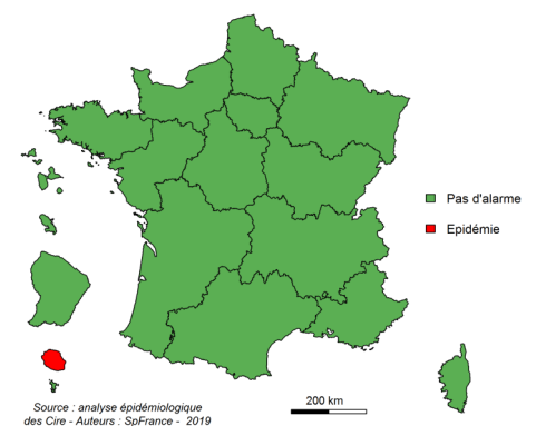
Figure 2 : Niveau d'alerte régional en semaine 43/2019
