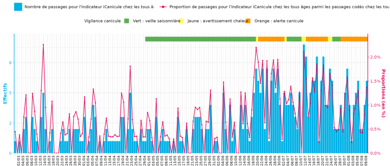
Figure 1. Nombre et proportions de passages aux urgences du réseau OSCOUR® pour iCanicule, tous âges et vigilance canicule départementale maximale observée, Corse, données au 11-08-2026
