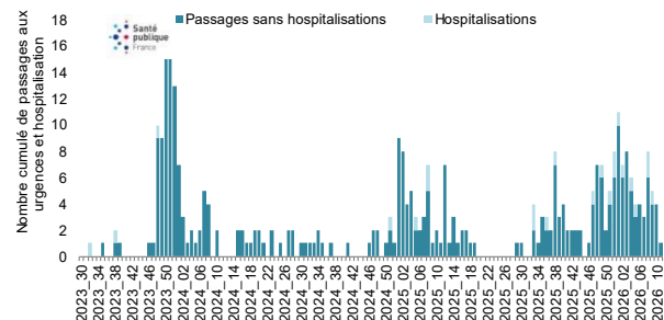
Figure 9 : Nombre hebdomadaire de passages aux urgences et hospitalisations pour syndromes grippaux - S2023-30 à S2026-11, Saint-Martin. Source Oscour®, exploitation Santé publique France
