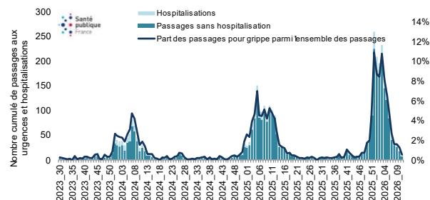
Figure 6 : Nombre hebdomadaire de passages aux urgences et hospitalisations pour syndromes grippaux - S2023-30 à S2026-11, Guadeloupe. Source Oscour® : exploitation Santé publique France
