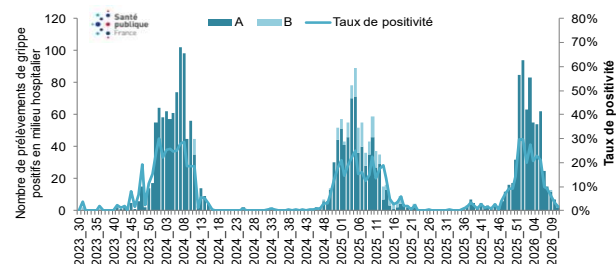
Figure 7 : Nombre hebdomadaire de résultats positifs au virus Influenza et taux de positivité - S2023-30 à S2026-11, Guadeloupe. Source : Laboratoire des Centres Hospitaliers de Guadeloupe, exploitation Santé publique France
