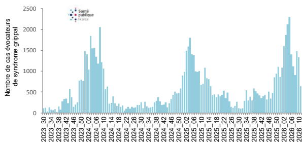
Figure 1. Nombre hebdomadaire de consultations pour syndromes grippaux en médecine de ville, Martinique - S2023-30 à S2026-11. Source : réseau de médecins sentinelles, exploitation Santé publique France
