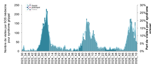
Figure 2. Nombre hebdomadaire de visites SOS Médecins pour syndromes grippaux, Martinique - S2023-30 à S2026-11. Source : SOS Médecins, exploitation Santé publique France
