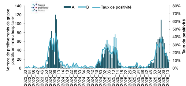
Figure 4 : Nombre hebdomadaire de résultats positifs au virus Influenza et taux de positivité - S2023-30 à S2026-11, Martinique. Source : Laboratoire de biologie du CHU de Martinique : exploitation Santé publique France
