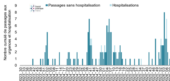
Figure 11 : Nombre hebdomadaire de passages aux urgences et hospitalisations pour syndromes grippaux - S2023-30 à S2026-11, Saint-Barthélemy. Source : Oscour®, exploitation Santé publique France
