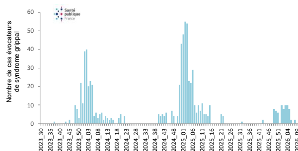
Figure 10. Nombre hebdomadaire de consultations pour syndromes grippaux en médecine de ville, Saint-Barthélemy - S2023-30 à S2026-11. Source : réseau de médecins sentinelles, exploitation Santé publique France
