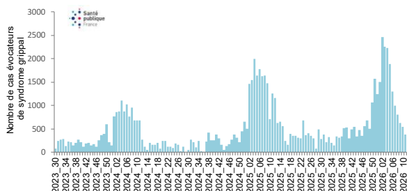
Figure 5. Nombre hebdomadaire de consultations pour syndromes grippaux en médecine de ville, Guadeloupe - S2023-30 à S2026-11. Source : réseau de médecins sentinelles, exploitation Santé publique France
