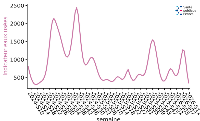
Figure 4 – Circulation du SARS-CoV-2 dans les eaux usées, de S08-2024 à S11-2026, en Corse (point au 17/03/2026)
