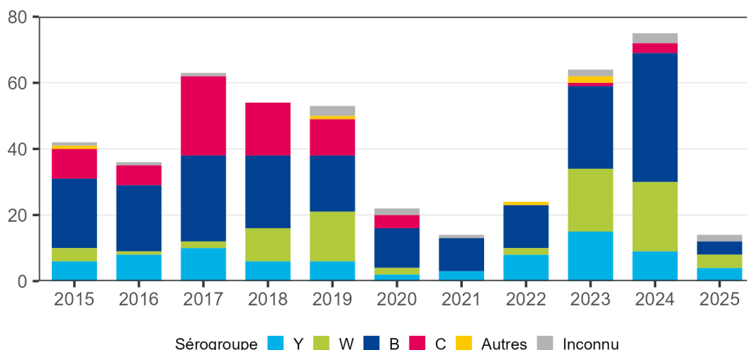
Figure 4. Nombre annuel de cas d'infection invasive à méningocoque domiciliés en Occitanie, selon le sérotype, janvier 2015 à mars 2025
