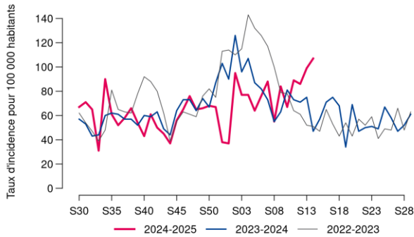
Figure 1. Taux d'incidence des consultations pour gastro-entérite aigüe réseau Sentinelles, tous âges, Occitanie
