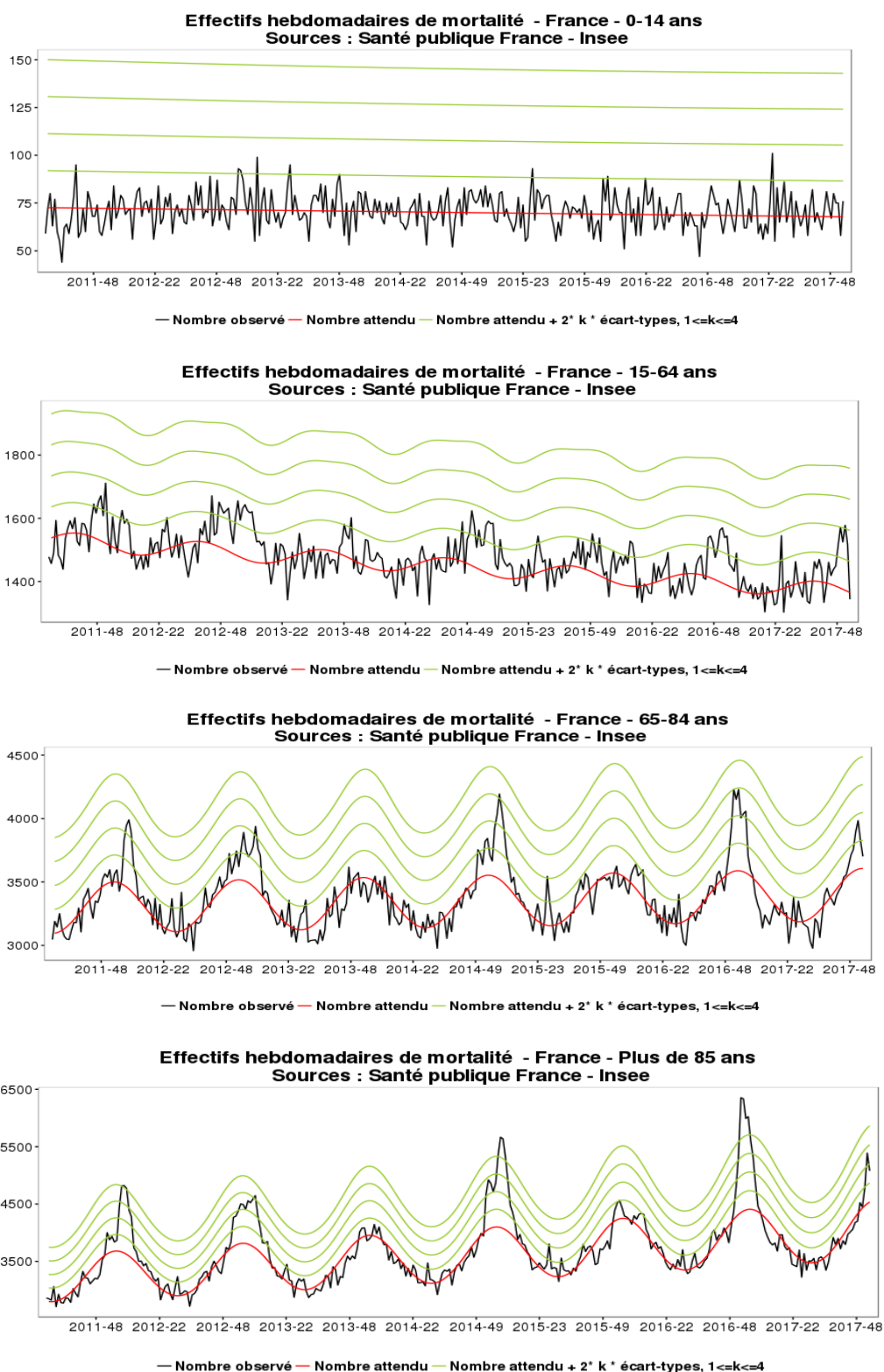
Fluctuations hebdomadaires de la mortalité par classe d'âges, 2011 à 2018 - France entière (effectif incomplet sur la dernière semaine) – Semaine 02-2018
