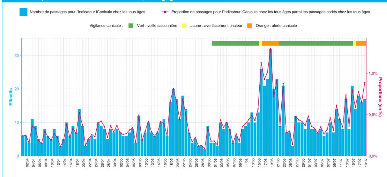
Figure 1. Nombre et proportions de passages aux urgences du réseau Oscour® pour iCanicule tous âges et vigilance canicule départementale maximale observée, Bourgogne-Franche-Comté, données au 20/07/2022
