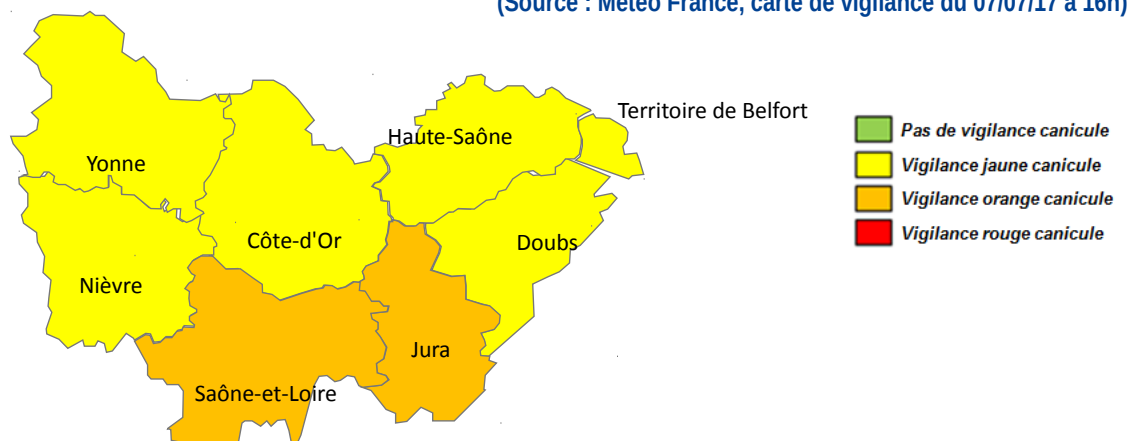
Figure 1 : Carte régionale des niveaux de vigilance canicule départementaux en région Bourgogne Franche-Comté (Source : Météo France, carte de vigilance du 07/07/17 à 16h)
